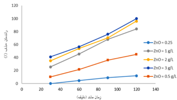
تصویر ۴. تأثیر غلظت نانوذرات اکسید روی بر حذف رنگ اسید بلاک یک در فرایند UV/H 2 O 2 /ZnO (ساعت ۲۱ الی ۴۱ ظهر، تابستان).
