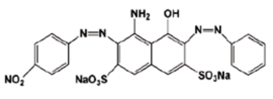
تصویر ۱. فرمول ساختاری رنگ اسید بلاک یک.
