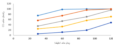
تصویر ۵. تأثیر غلظت اولیه رنگ اسید بلاک یک بر عملکرد حذف فرایند UV/H 2 O 2 /ZnO (ساعت ۲۱ الی ۴۱ ظهر، تابستان).
