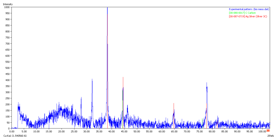
شکل ۳. الگوی XRD نانوذرات نقره سنتز شده با زیست توده. پیک در زاویه‌های ۰/۲۲، ۳۸/۴۱، ۴۴/۵۱، ۵۱/۶۰، ۷۶/۱۷ و ۷۷/۸۰ مربوط به کریستال‌های نقره که به رنگ قرمز مشخص شده است.
