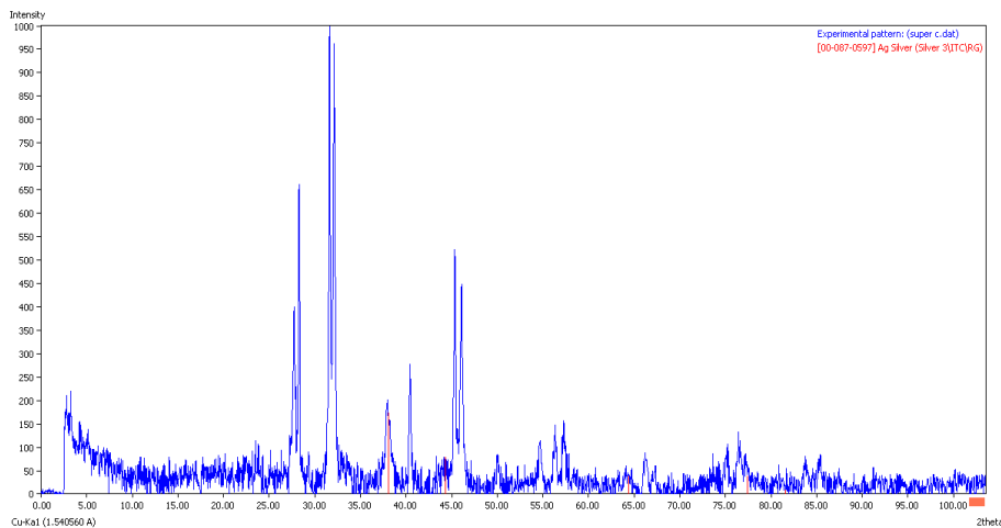
شکل ۲. الگوی XRD نانوذرات نقره سنتز شده با سوپرناتانت. پیک در زاویه‌های ۰/۵، ۳۸/۰۵، ۴۴/۳۴، ۴۴/۴۹، ۶۴/۳۶ و ۸۱/۴۷ مربوط به کریستال‌های نقره که به رنگ قرمز مشخص شده است.
