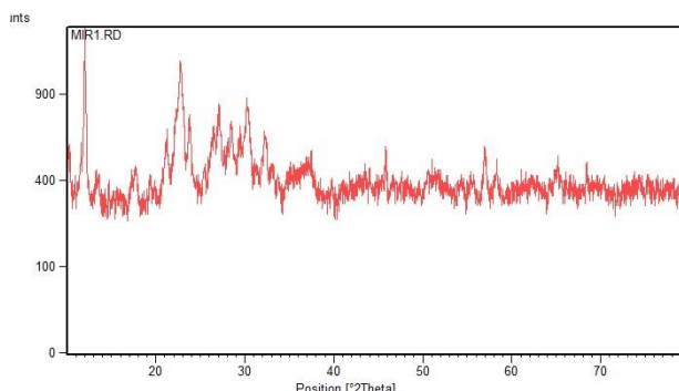
شکل ۱. آنالیز پراش اشعه ایکس زئولیت کلینوپتیلولولایت
