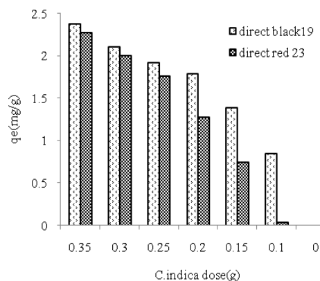
شکل ۵: تأثیر دوزهای مختلف بیومس سیتوسیرا ایندیکا بر حذف رنگ مشکی و قرمز مستقیم (غلظت اولیه هریک از ترکیبات رنگی ۲۰ mg/L، زمان تماس ۱۲۰ دقیقه و pH=۵)
